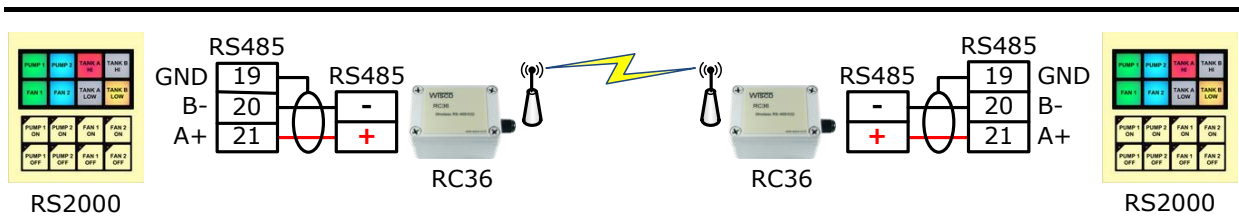
การเชื่อมต่อระหว่าง RS2000 กับ DIO2100 ผ่านทาง Wireless (RC36)
