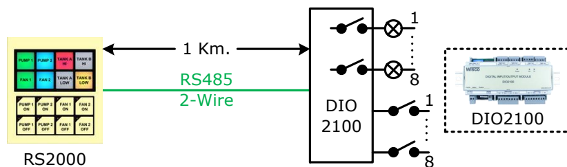
การต่อใช้งานร่วมกับ DIO2100 ผ่านทาง RS485
