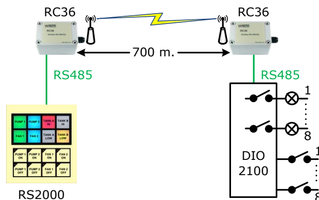
การต่อใช้งานร่วมกับ Wireless (RC36) ผ่านทาง RS485
