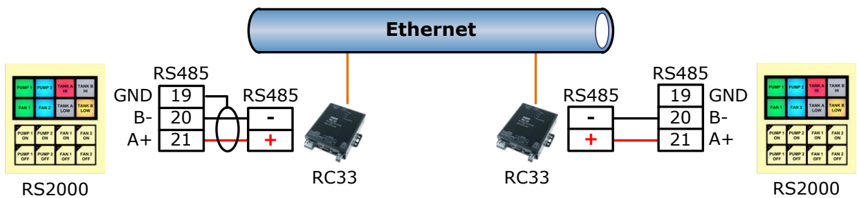
การเชื่อมต่อระหว่าง RS2000 กับ DIO2100 ผ่านทาง Network (LAN)
