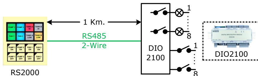
การต่อใช้งานร่วมกับ DIO2100 ผ่านทาง RS485
